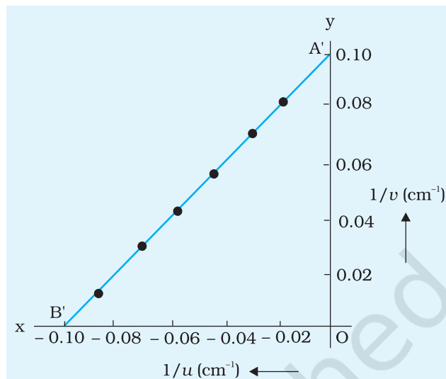
चित्र E 10.5 1/u तथा 1/v के बीच सरल रेखीय ग्राफ (पैमाने के अनुसार नहीं)
