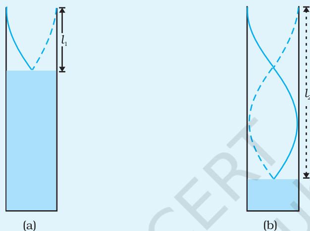
चित्र E 16.2 अनुनाद नली में कंपन
